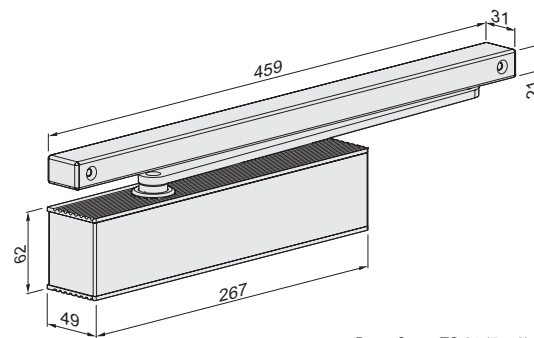
Bemaßung: TS-61 (5 – 6)
