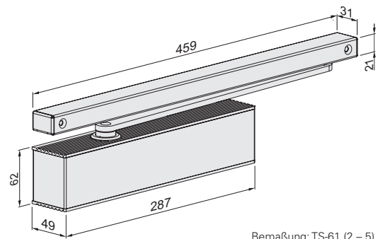
Bemaßung: TS-61 (2 – 5)
